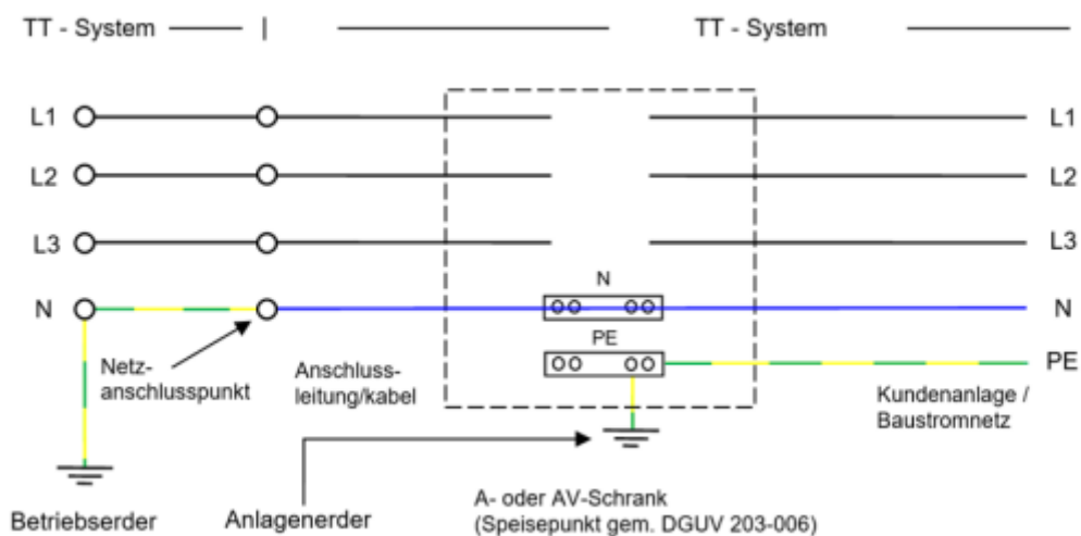
Abbildung 6 Anschlussmöglichkeiten am Beispiel des TT-System
